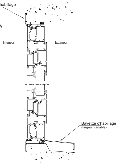
Coupe A-A
